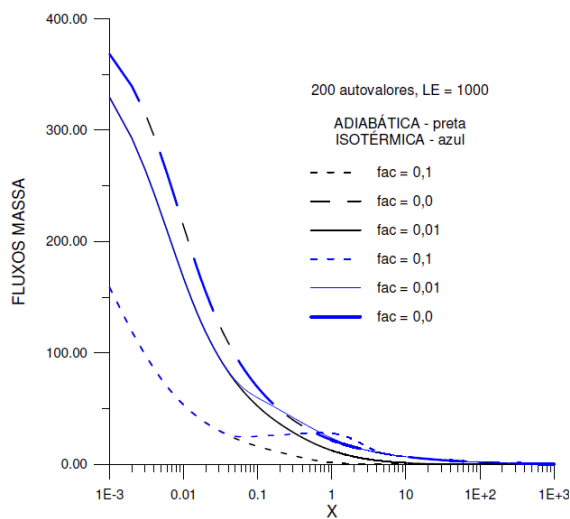
Fig. 7. Fluxo de massa na interface para parede adiabática isotérmica.
