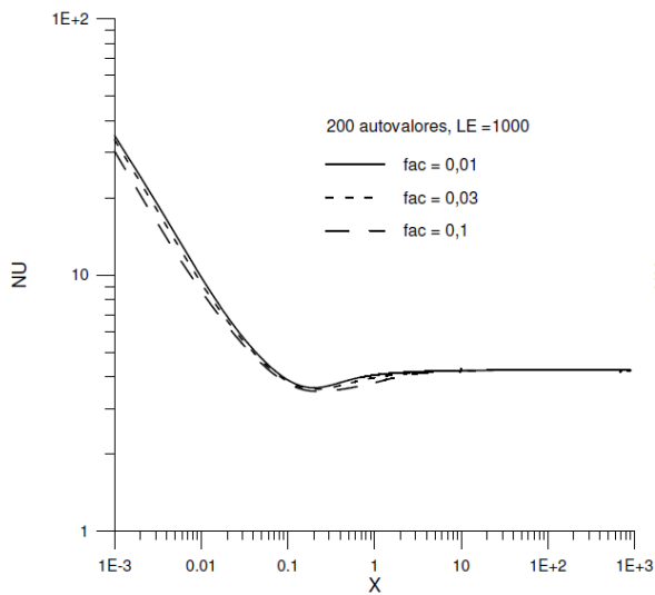
a) Interface (parede isotérmica)
