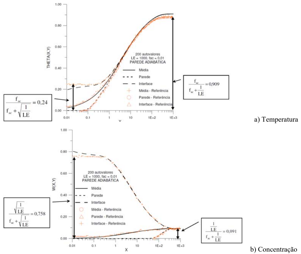
Fig. 2. Comparação da distribuição de temperatura e concentração em relação aos resultados da referência para paredes adiabáticas.
