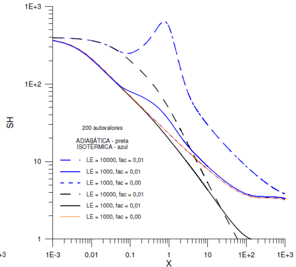
Fig. 8. Número de Sherwood para condições de parede e adiabática e isotérmica).
