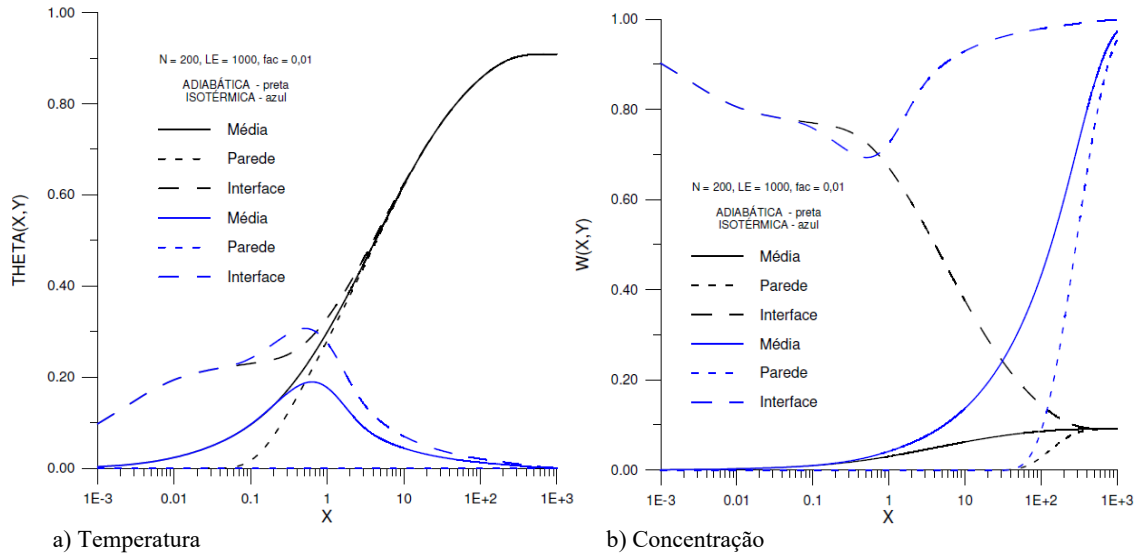
Fig. 4. Comportamento da distribuição de temperatura e concentração para parede adiabática e isotérmica.
