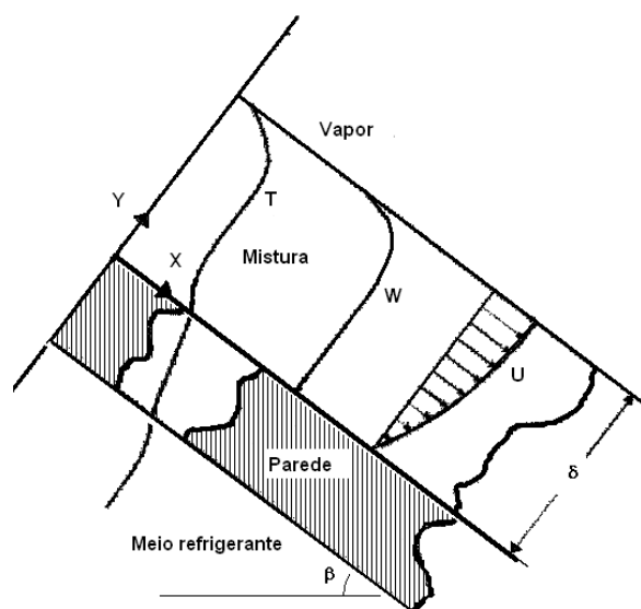
Fig. 1. Escoamento da película absorvente sobre uma placa inclinada com espessura constante.
