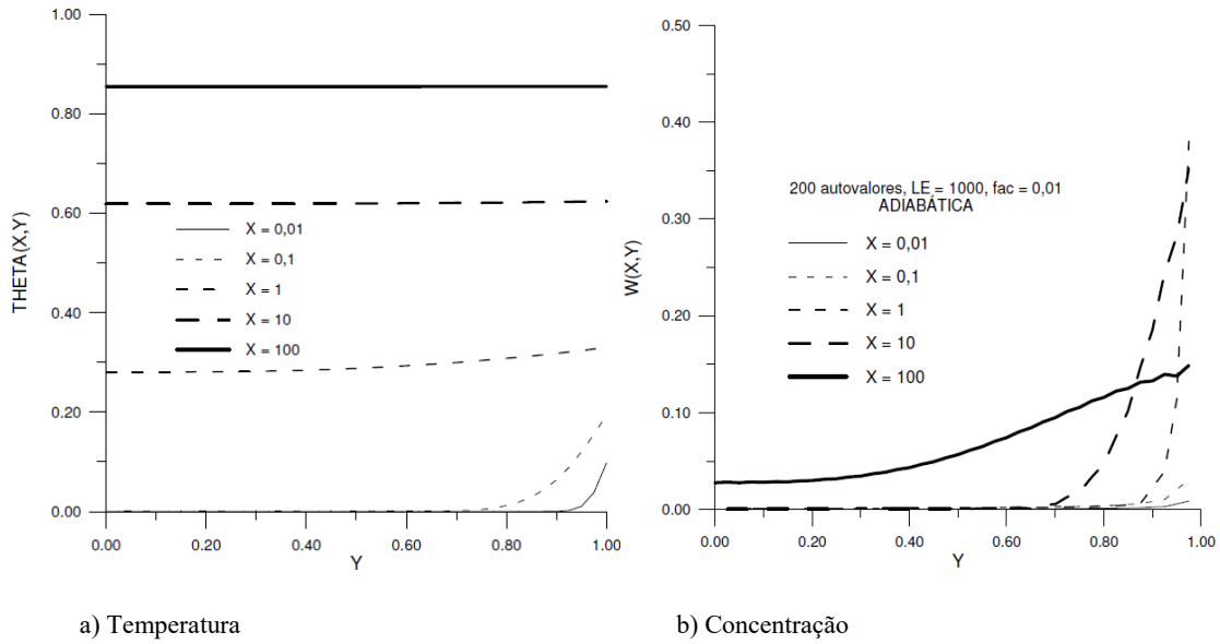
Fig. 5. Perfis de temperatura e concentração para diferentes valores de X com Le = 100 e fac = 0,01 (parede adiabática, 200 autovalores).
