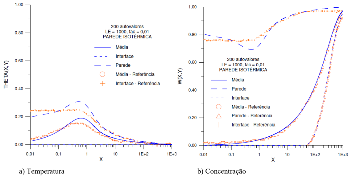
Fig. 3. Comparação da distribuição de temperatura e concentração em relação aos resultados da referência para paredes isotérmicas.
