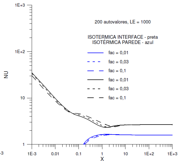
b) Interface e parede (parede adiabática)
