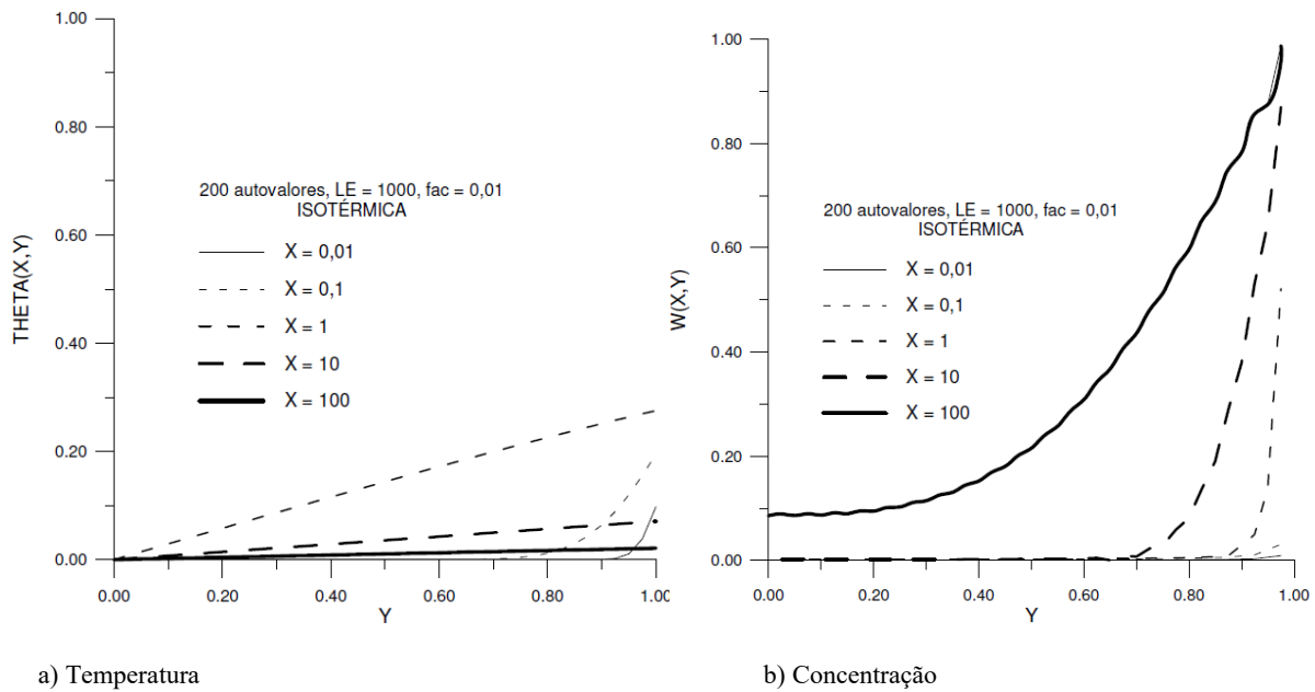
Fig. 6. Perfis de temperatura e concentração para diferentes valores de X com Le = 100 e fac = 0,01 (parede isotérmica, 200 autovalores).
